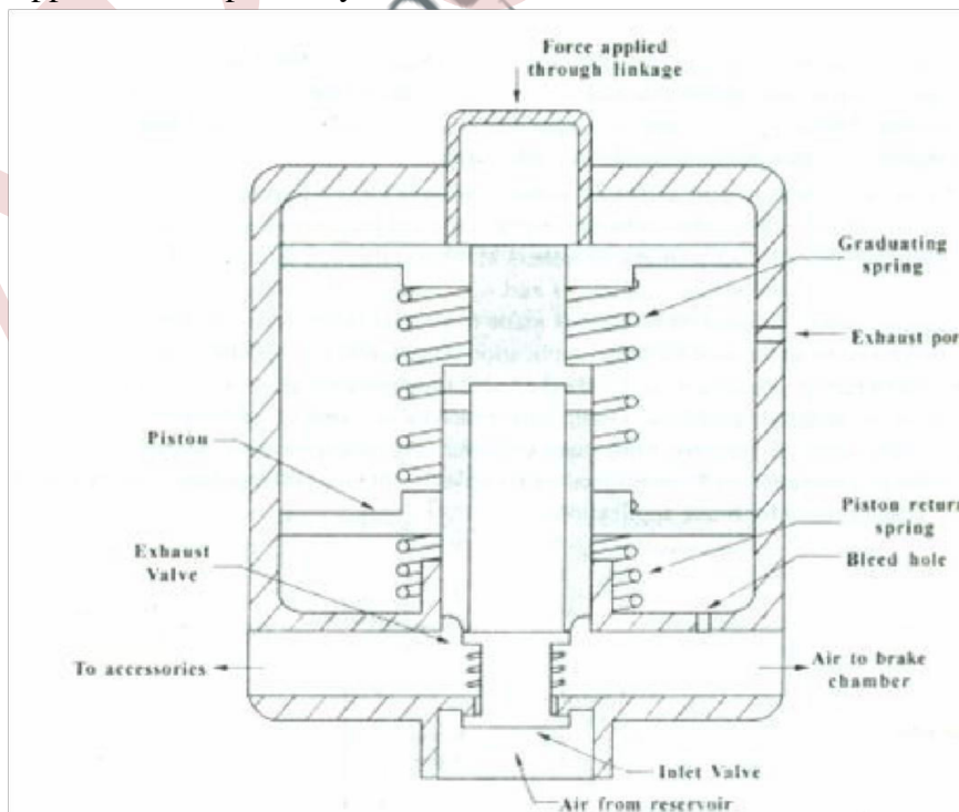
Fig: Brake valve
