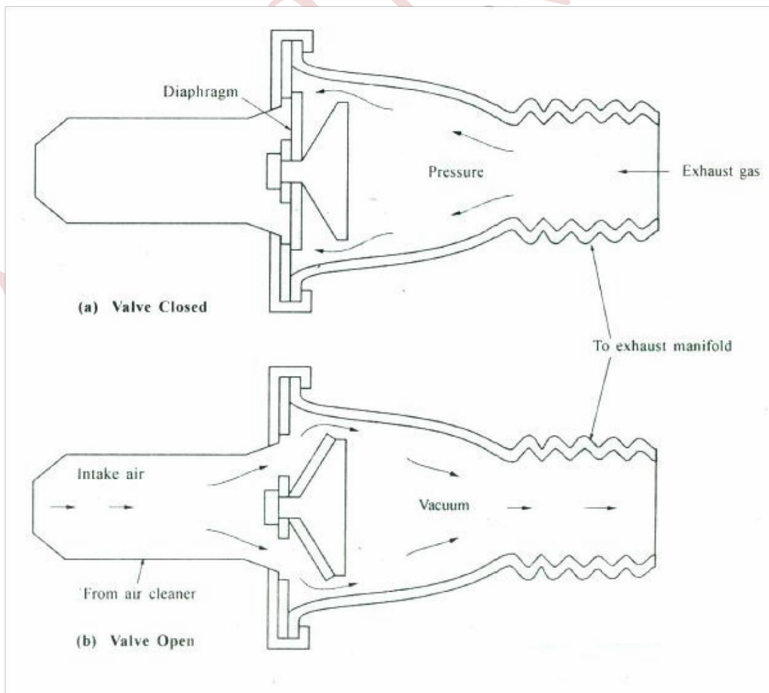
Fig: Air aspirator valve
