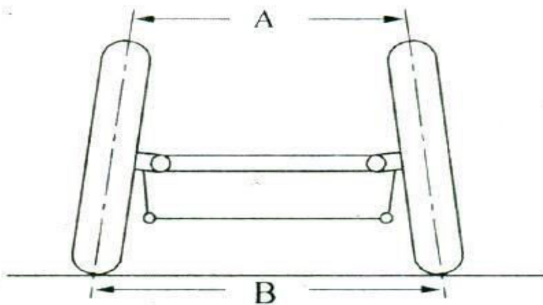
Fig: Toe - in
