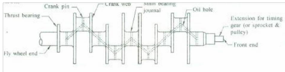
Fig: Crank Shaft
