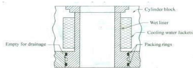
Fig: Wet liners
