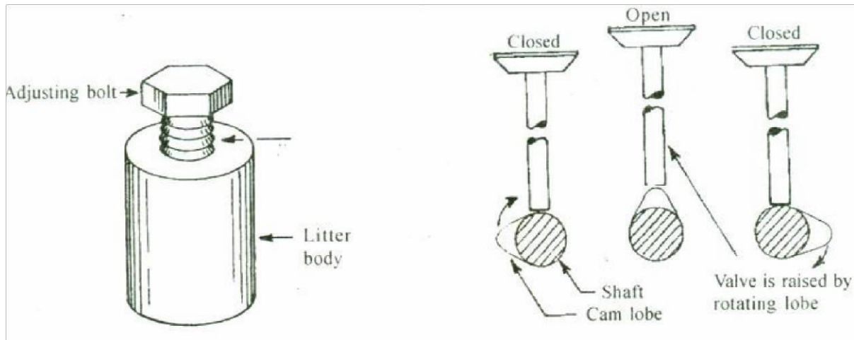
Fig: (e) Valve lifter
