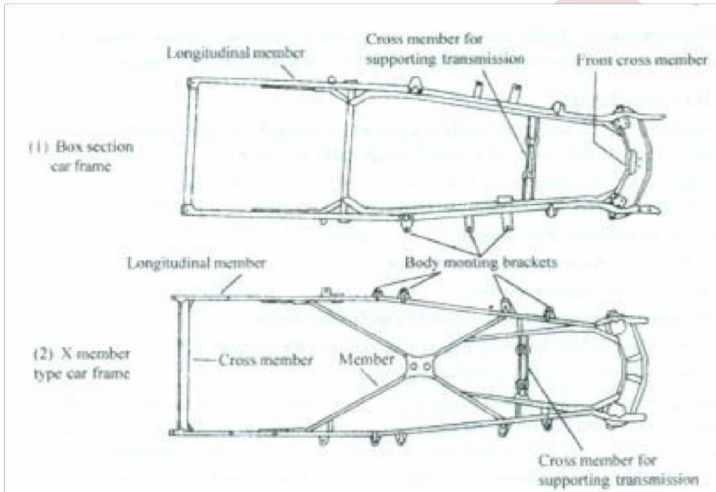
Fig: Chassis Frame
