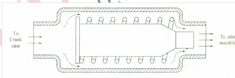
Fig: PCV Valve
