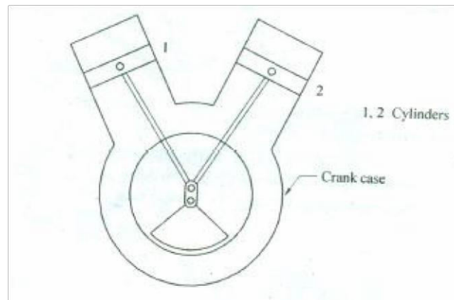
Fig: V-engine
