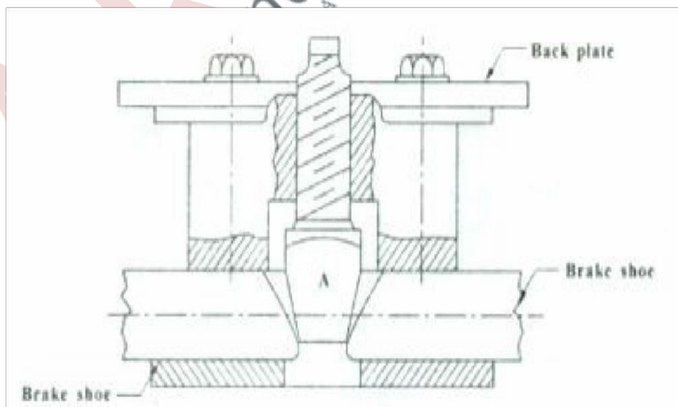
Fig: Expander
