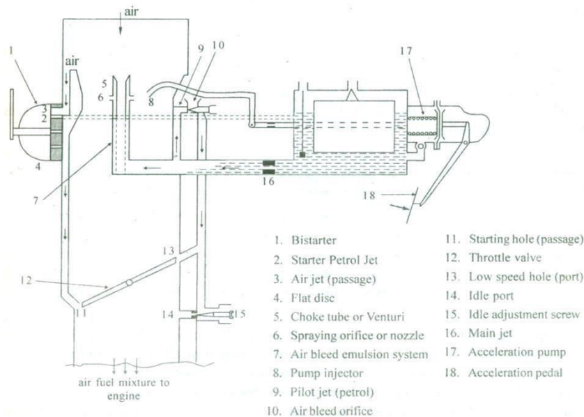
Fig: Solex Carburetor
