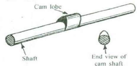
Fig: (d) Cam shaft valve mechanism
