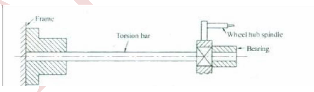
Fig: Torsion bars
