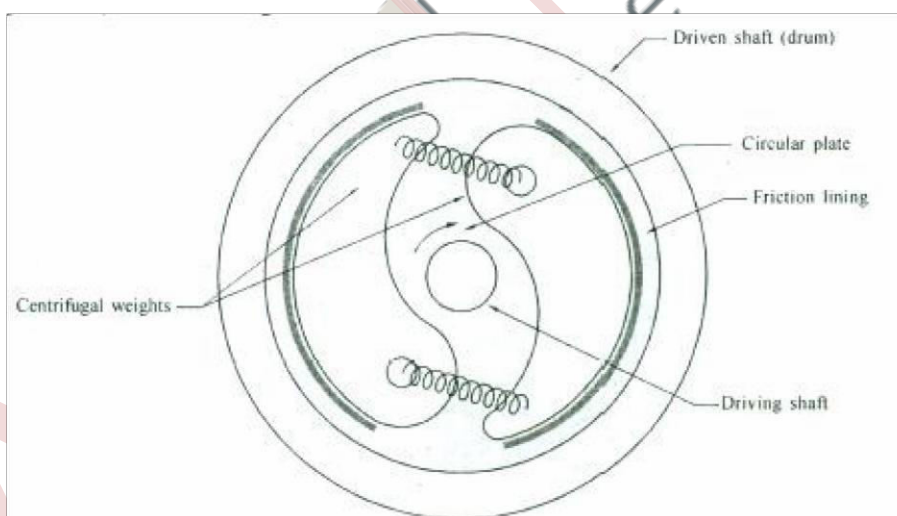
Fig. Centrifugal Clutch
