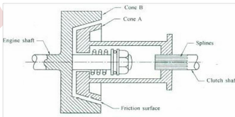
Fig: Cone clutch
