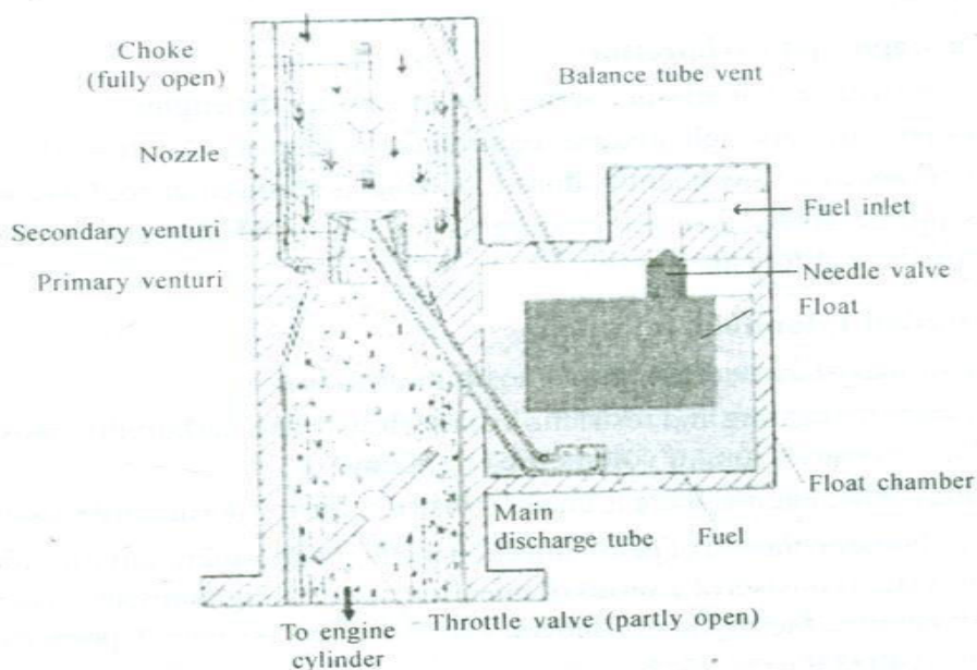
Fig: Simple Carburetor
