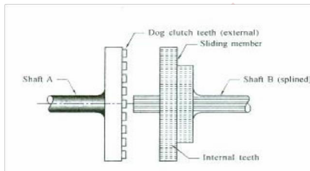
Fig. Dog Clutch
