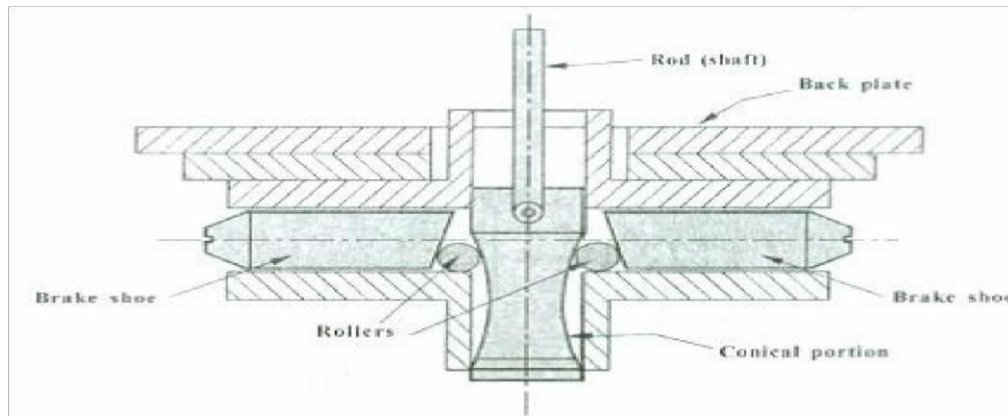
Fig: Adjuster
